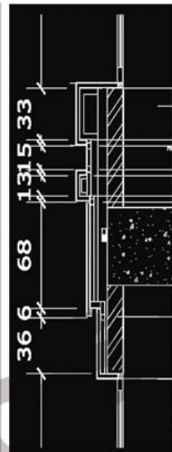
نقشه های کارگاهی و اجرایی
